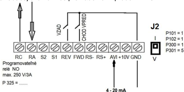
Príklad zapojenia ovládacej svorkovnice pre riadenie fr. prúdom 4-20 mA:
